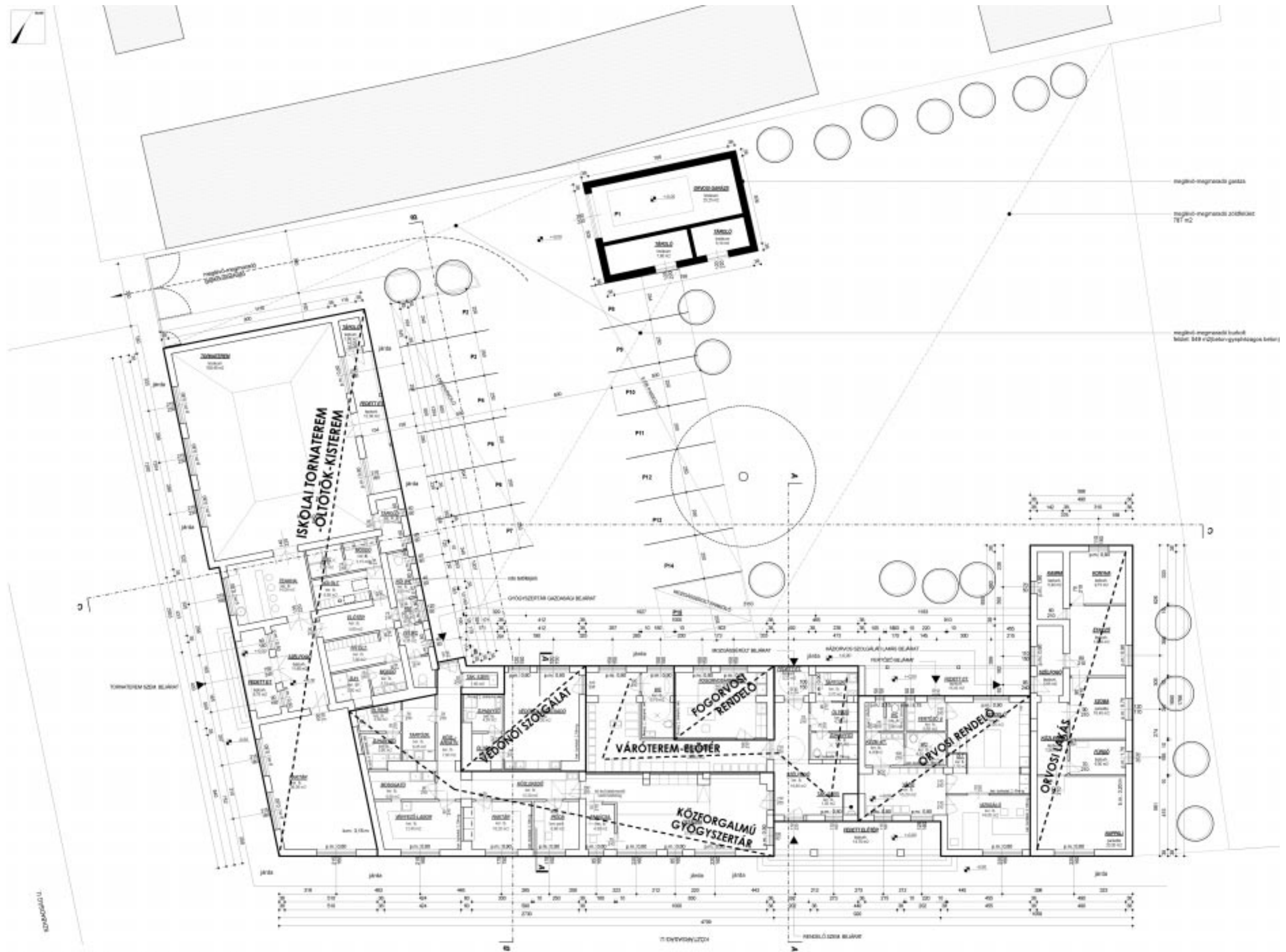
ALAPRAJZ M1:100 - 2010. SZEPTEMBER
